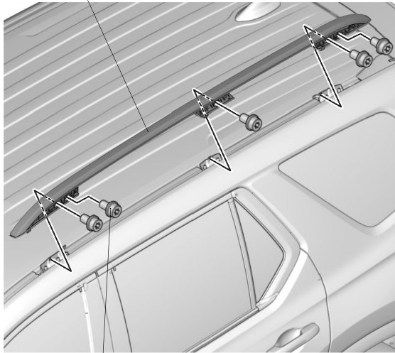
5 TORX BOLTS
